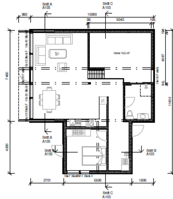
2.0 - Hems 1:100
