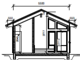
Snitt B 1 : 100
