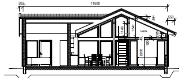
Snitt C 1 : 100
