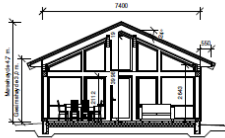
Snitt A 1 : 100
