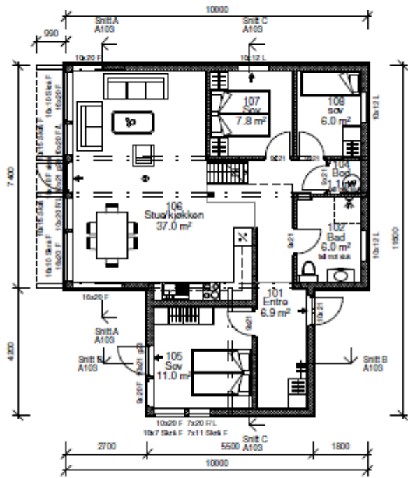
1.0 - 1. Etasje 1:100
