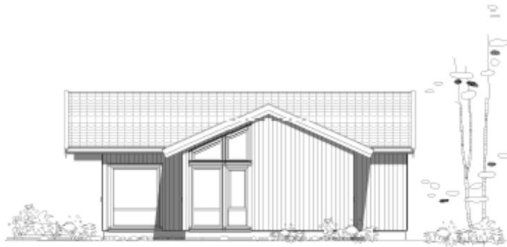
Fasade mot sør-vest 1 : 100
